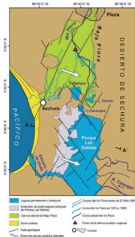
Figura 3. Mapa de los desplazamientos laterales del sistema fluvial del Bajo Piura y del sistema lacustre temporal de pampa Las Salinas, en el contexto de fallas geológicas identificadas en el análisis morfo-estructural de datos de teledetección (Rajchl et al., 2010). Se muestran desplazamientos del río y del borde occidental de la laguna temporal hacia el este. Es evidente la influencia de las fallas en la geometría y la evolución de ambos sistemas sedimentarios. Las flechas indican la dirección de los desplazamientos. Las marcas negras delimitan la línea del perfil topográfico A-A' de la figura 4
