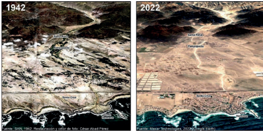
Figura 3. Cono de deyección del torrente Malanche en los años 1942 y 2002
