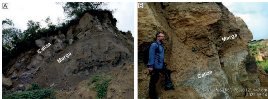
Figura 3. Alternancia de calizas masivas micríticas y biomicríticas con capas de margas de la formación Cajamarca (A, B).
